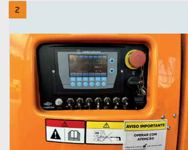
2 Caixa de controle da base: a caixa de controle pode ser usada para controlar cada ação do dispositivo, de fácil compreensão
