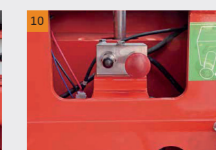
Válvula de liberação manual: Quando a máquina não puder se mover, você pode empurrar a máquina depois de pressionar esta válvula
